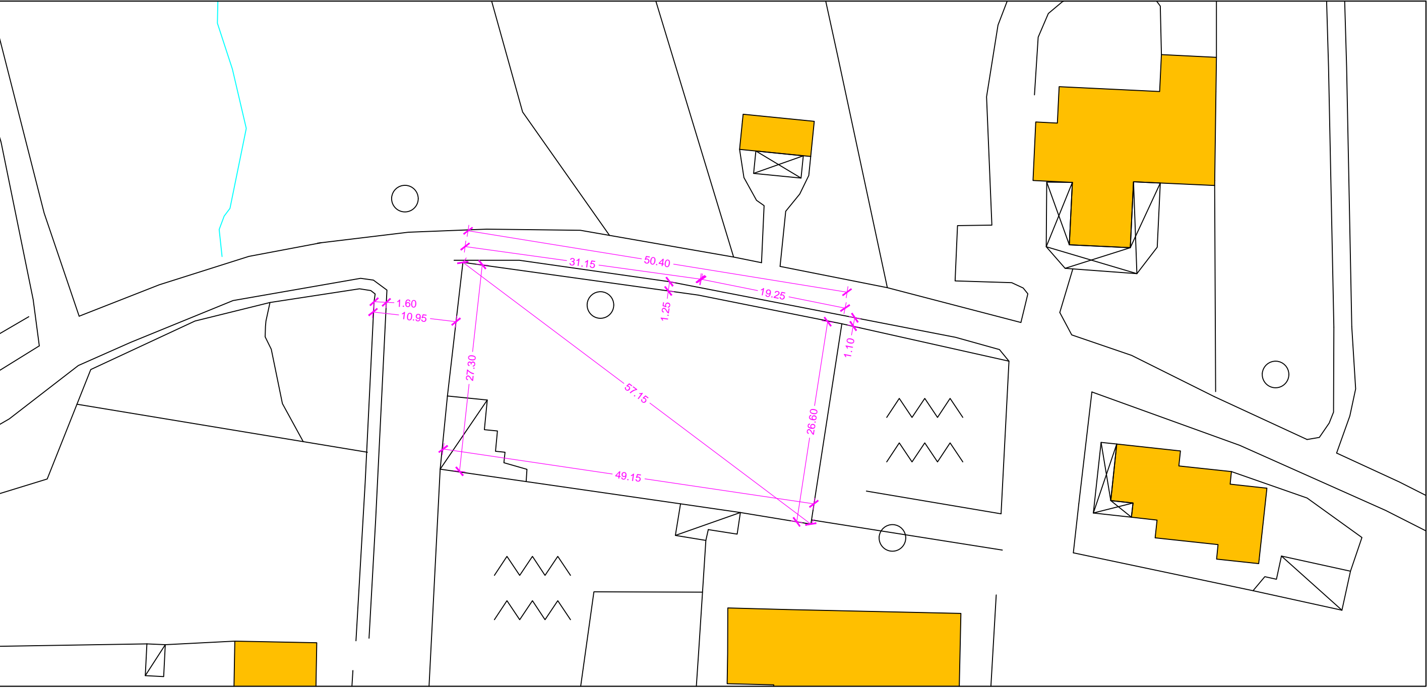
RILIEVO CELERIMETRICO 1:500
